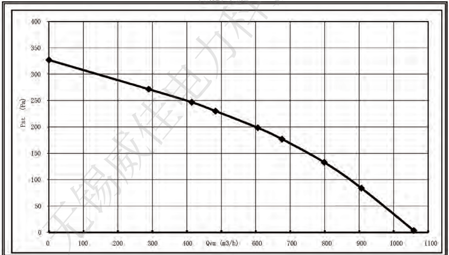
性能曲线
