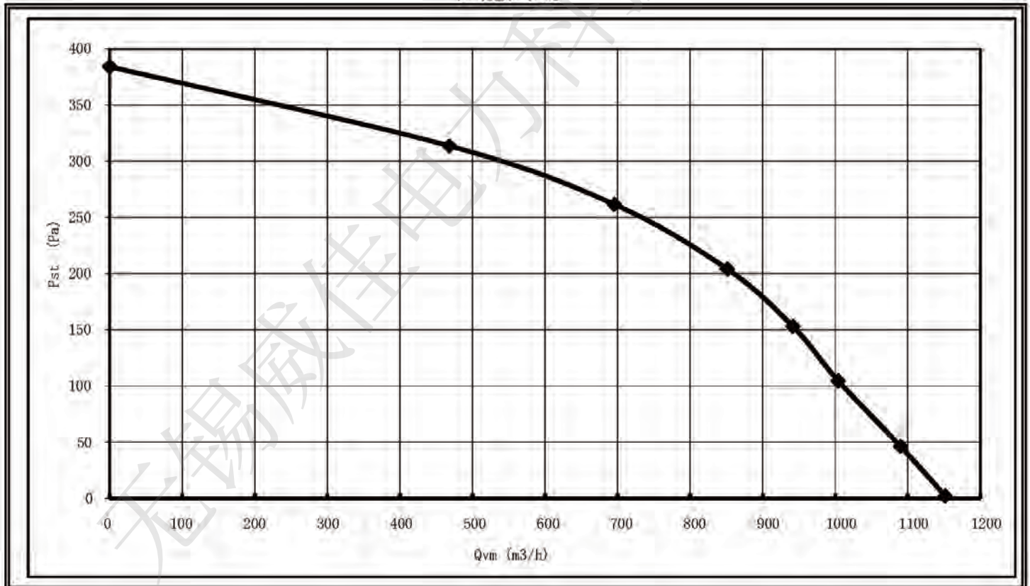
性能曲线
